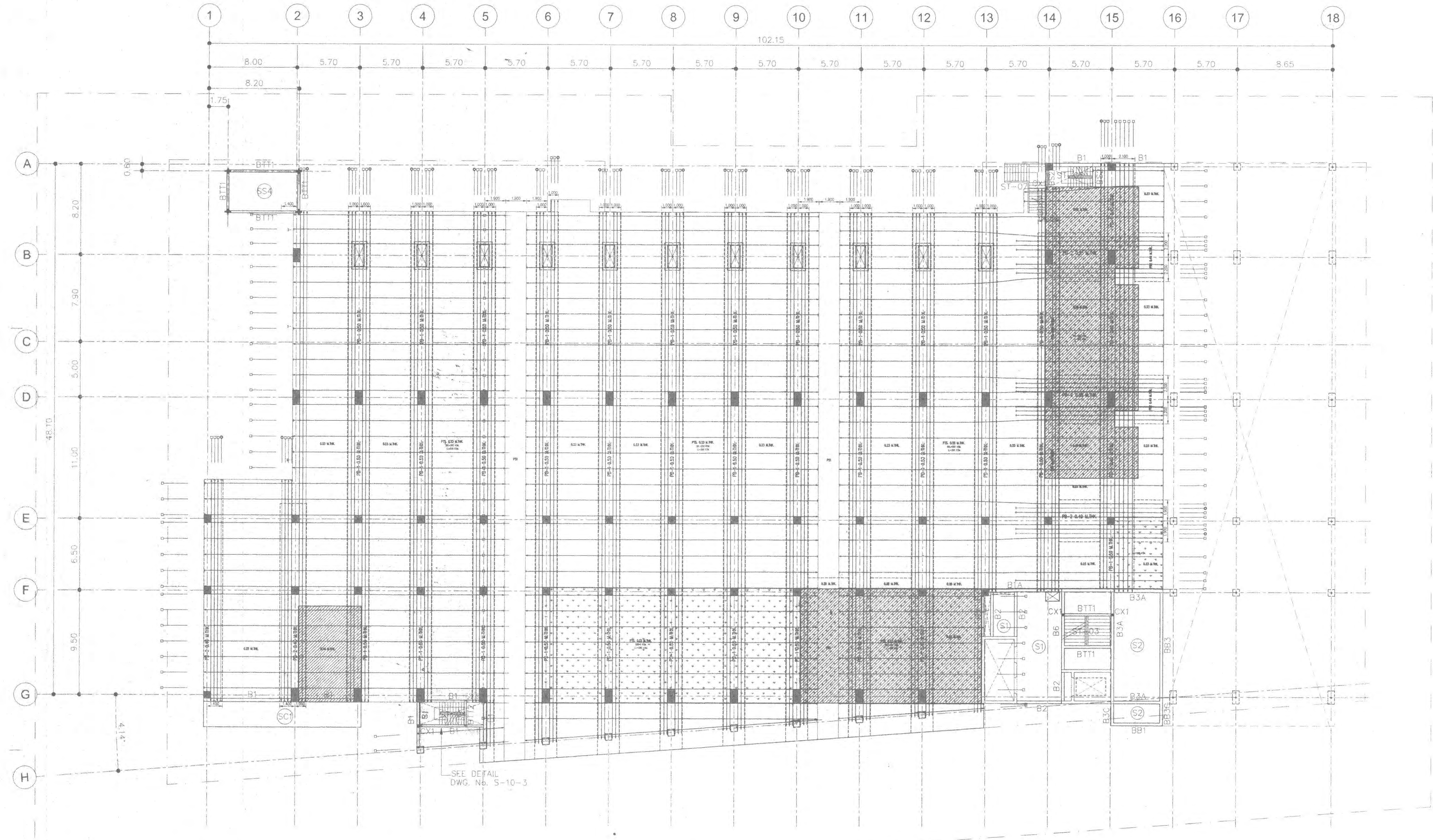
แปลนพื้นชั้น 2 (TENDON LAYOUT) 1:200
